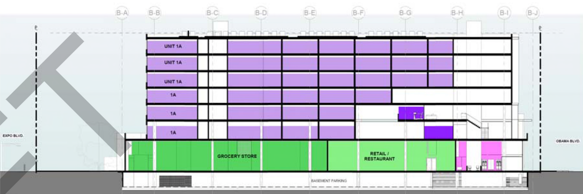
CROSS SECTION D - D'
