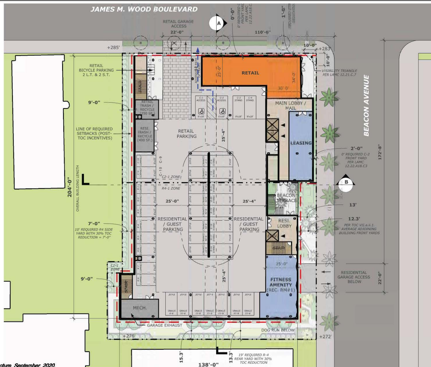
PROJECT SITE PLAN (LEVEL 2)
